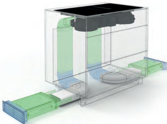
U5 Umluft mit Ausblasgittern, seitlich liegender Umluftfilter
