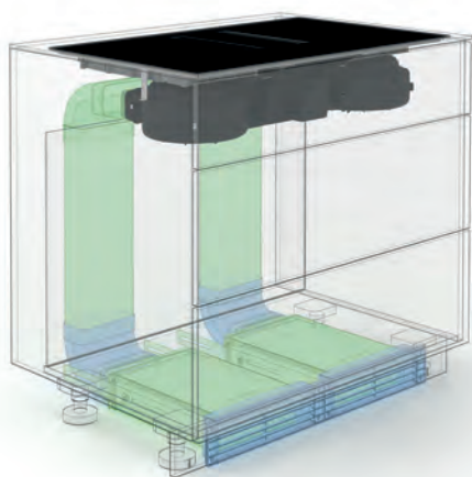
U4 Umluft mit Ausblasgittern, vorne liegender Umluftfilter
