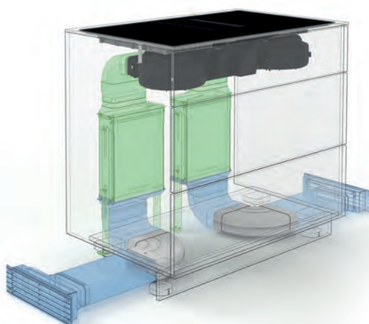
U3 Umluft mit Ausblasgittern, seitlich stehender Umluftfilter
