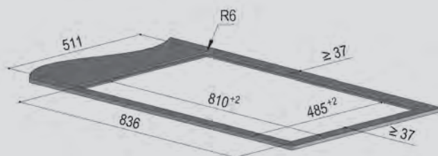
flächenbündiger Einbau
