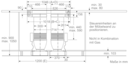
Kombination 2x Lüftungselemente 1x Kochfeld 80 cm
