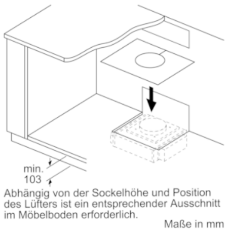
Ansicht Luftauslass
