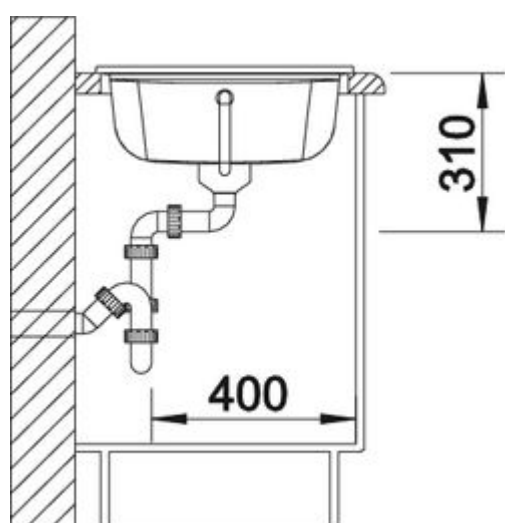
Seitenansicht
