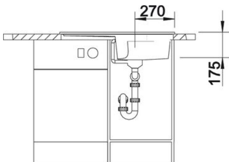
Frontansicht
