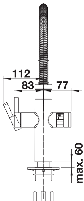
Seitenansicht Hebel
